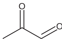
Methylglyoxal
